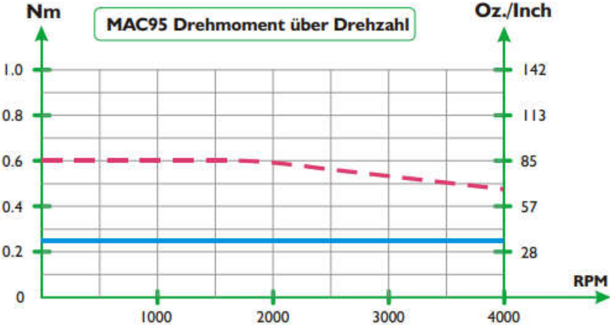
Drehmoment/Drehzahl-Kennlinie
